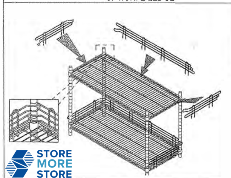
OPTIONAL LEDGE
