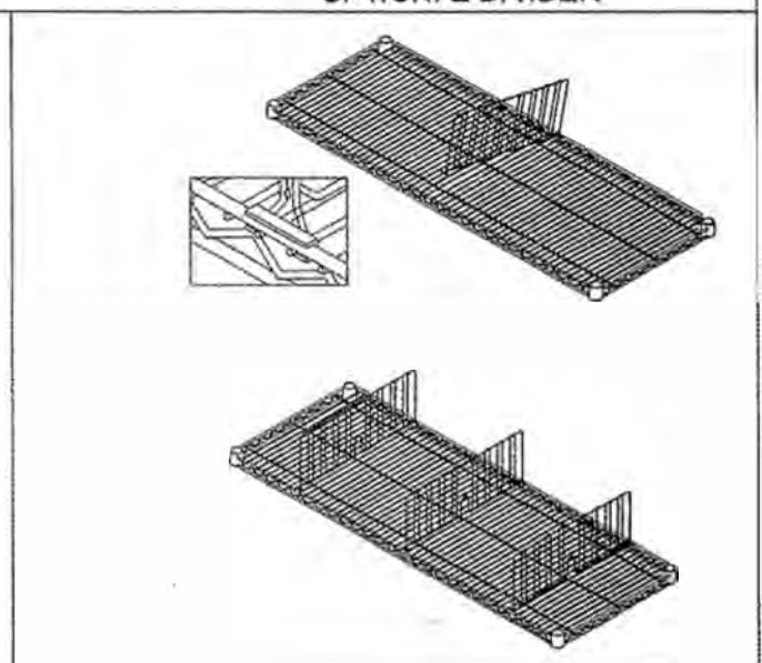
OPTIONAL DIVIDER
